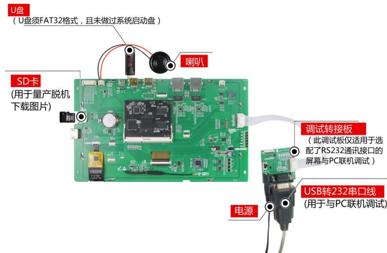
图 1-3 调试工具图
