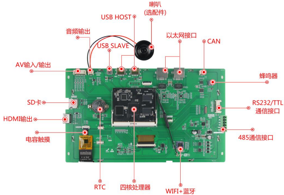
图 1-2 硬件配置图
